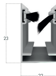
Section coulisse basse
