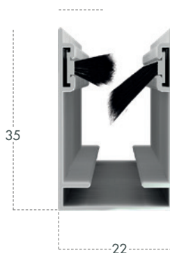
Section coulisse haute
