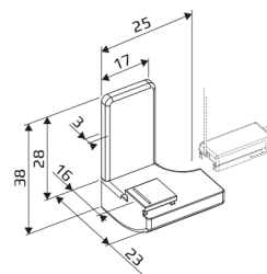
Équerre
