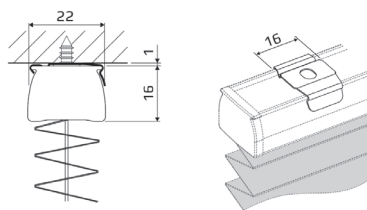
Pose plafond
